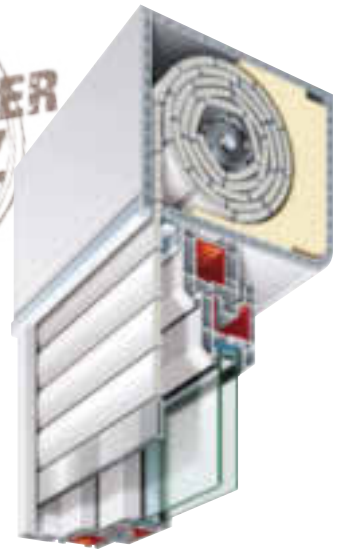
Aufsatzrollladen, Alu-Serie AAL * Rollläden mit Aufsatzkasten und Aluminium-Panzer, Standardfarbe Weiß, Kasten und Führungsschienen aus Kunststoff, Aluminium-Panzer, ausgeschäumte Alu-Profilen, inkl. Gurtbetrieb, Beispiel 1-tlg. Ausführung, Maße 900 x 900 mm (BxH) ab 239.99
