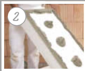
2 Polystyrol-Hartschaumplatte verkleben
