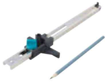
Laminat-Einpasser Ausmessen und Übertragen der letzten Laminatreihe, Art.-Nr. 1150322 12.99
