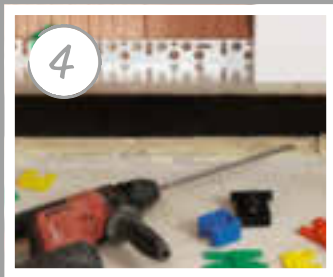
4 Sockelabschlussprofil anbringen
