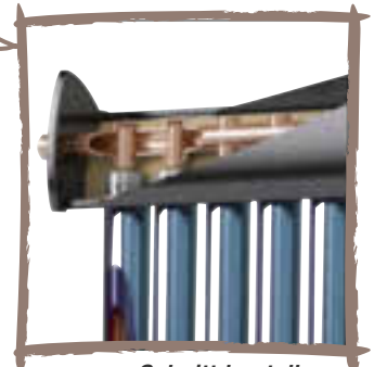
Schnittdarstellung BHP-Röhrenkollektor
