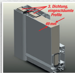
Aluminium-Mehrkammerprofil
