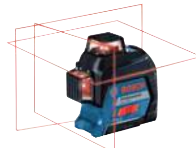
Linienlaser „GLL 3-80“ Professional horizontale und vertikale Nivellierarbeiten durch 3x360°-Laserlinien, Arbeitsbereich bis zu 30 m, Art.-Nr. 1490333
