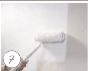
7 Putzgrundierung vorstreichen
