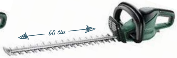
Elektro-Heckenschere „UniversalHedgeCut 60“ *** 420 Watt, Messerlänge 60 cm, Zahnöffnung 30 mm, Art.-Nr. 4101330 169.99*
