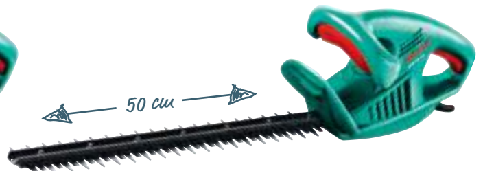
Elektro-Heckenschere „AHS 50-16“ *** 450-W-Motor, Messerabstand 16 mm, Art.-Nr. 4100044 79.99*
