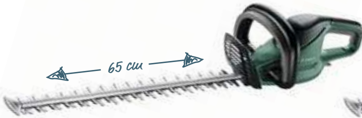
Elektro-Heckenschere „AdvancedHedgeCut 65“ *** 450 Watt, Messerlänge 65 cm, Zahnöffnung 34 mm, Art.-Nr. 4101331 189.99*
