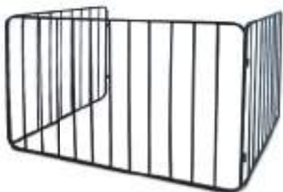
Sicherheitsgitter 3-teilig, schwarz, beschichtet, 74 cm (H), Seitenteile 84 cm (B), Mittelteil 112 cm (B), Art.-Nr. 3200200
